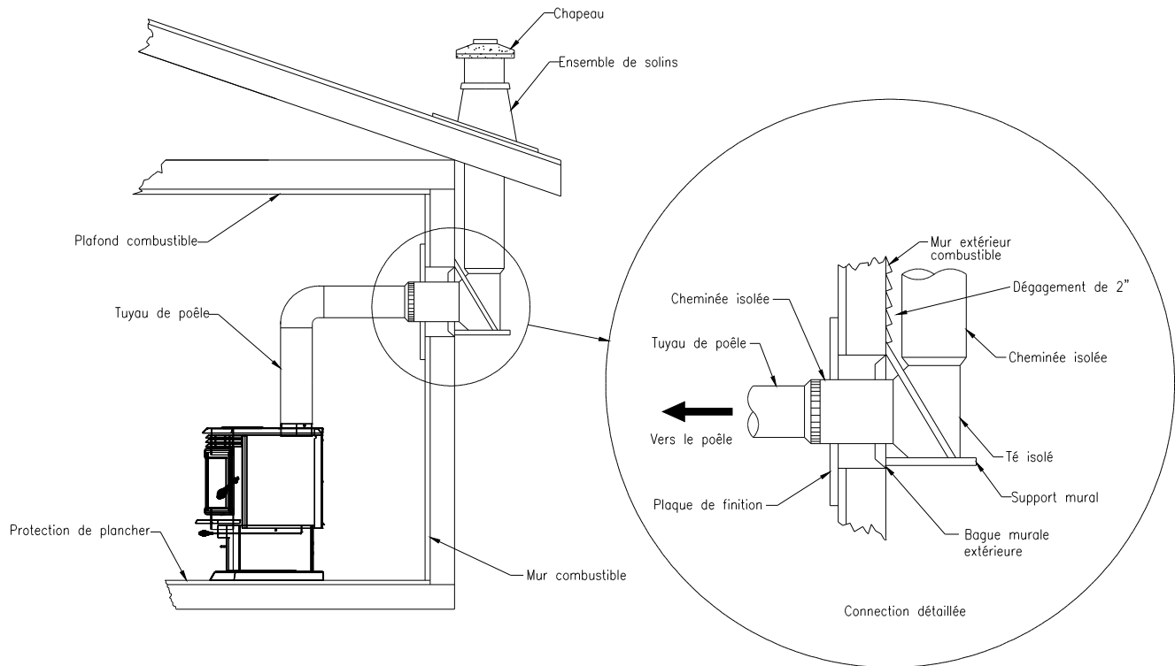
FIGURE 2.2.1 (A) Installation à travers le mur
