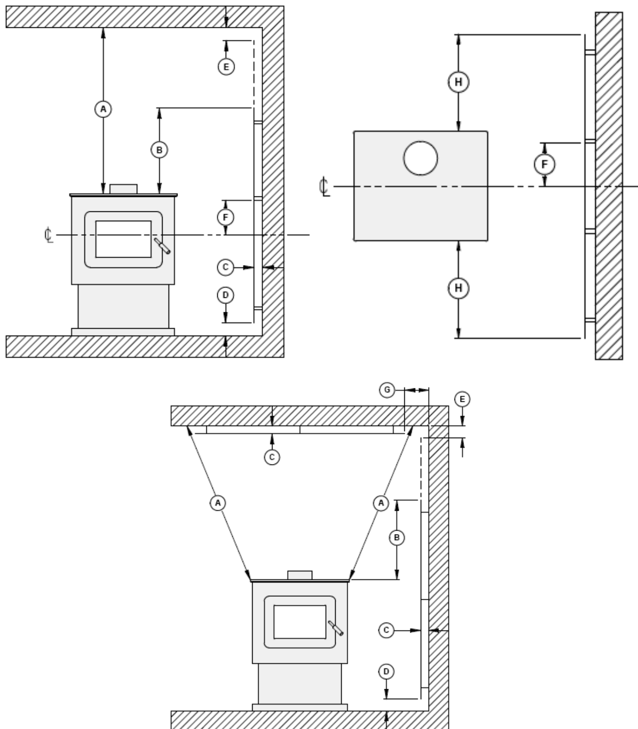
Dégagements pour construction de l'écran
