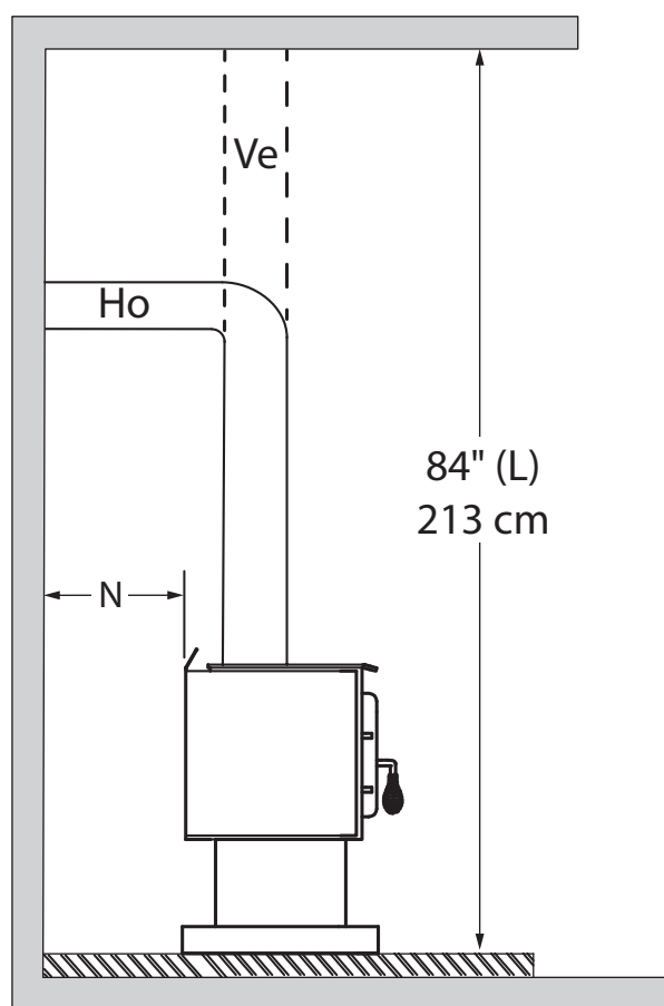
Figure 18: Dégage-ments - Côté
