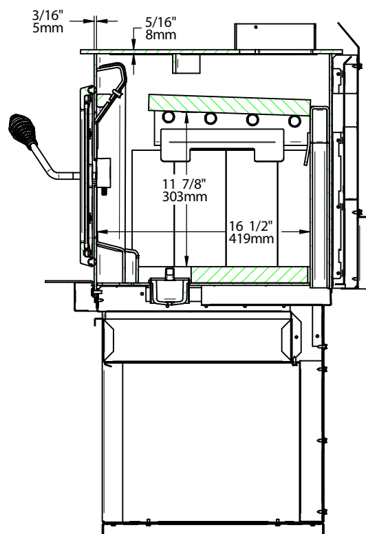
Figure 6: Vue de côté - chambre à combustion
