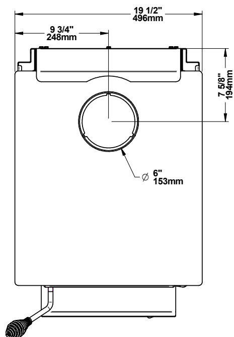
Figure 1: Vue de dessus
