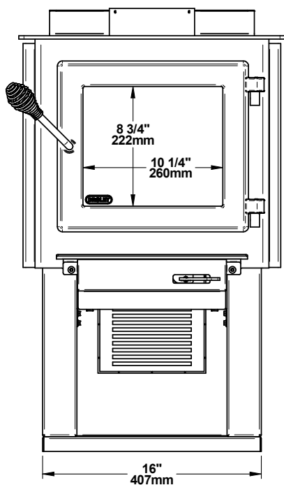
Figure 2: Vue de face
