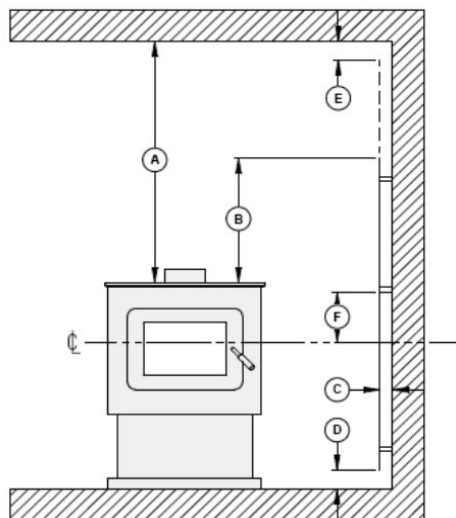
Figure 17: Dégagements pour l'écran de chaleur
