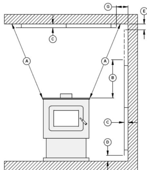
Figure 18: Dégagements pour l'écran de chaleur
