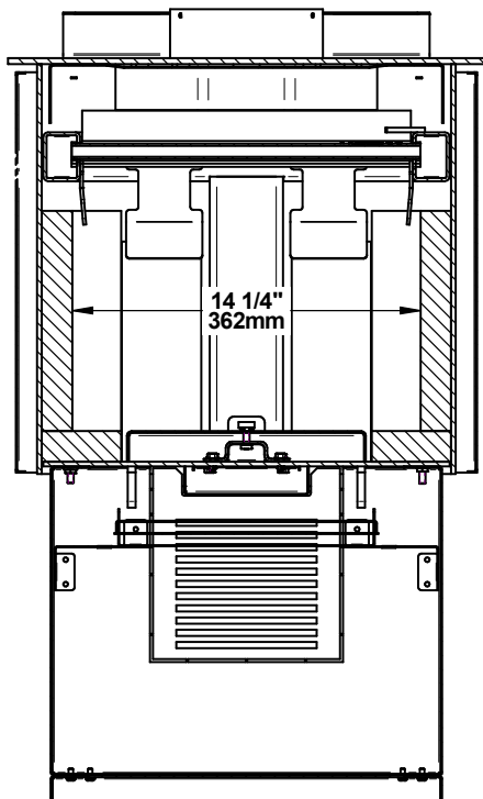
Figure 5: Vue de face - chambre à combustion
