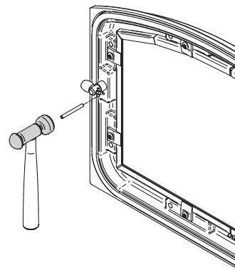
Figure 22: Installation de la goupille de retenue
