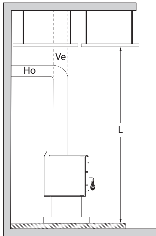
Figure 12: Dégagements - Plafond
