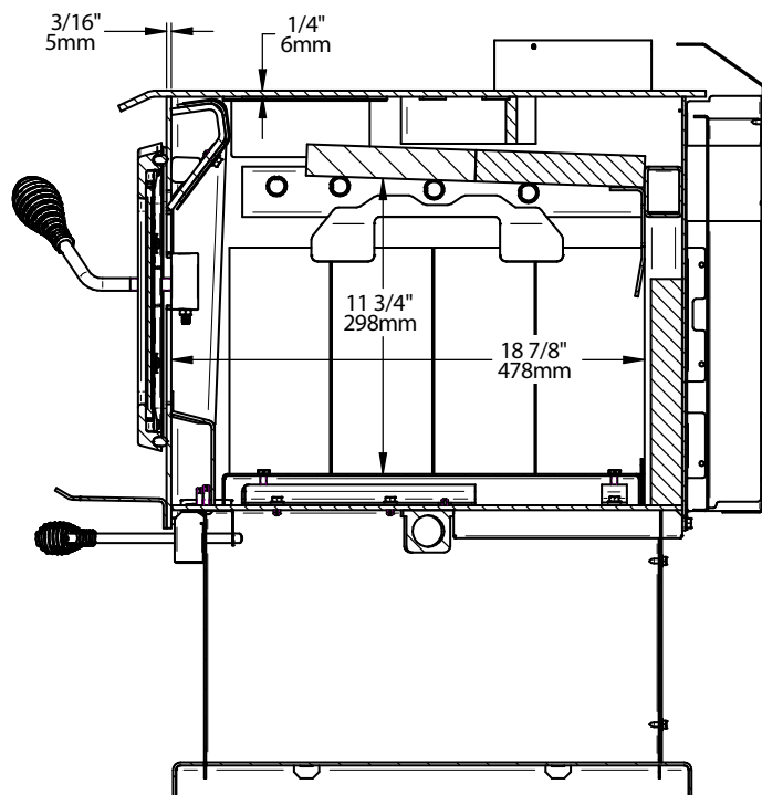
Figure 6: Vue de côté - chambre à combustion
