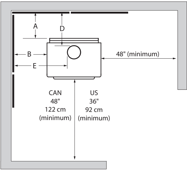
Figure 10: Dégagements - Vue dessus avec écran
