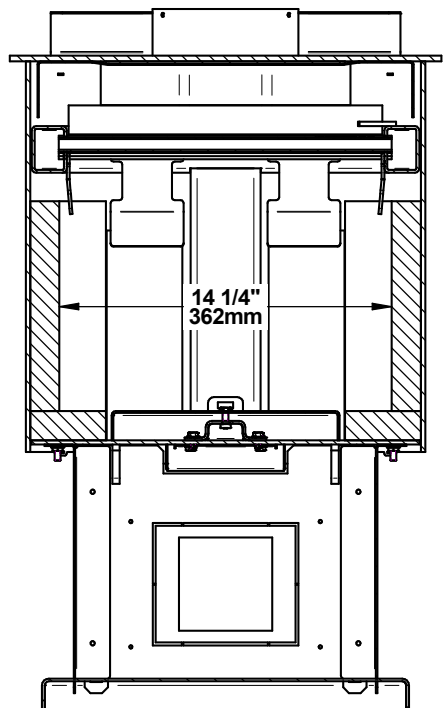
Figure 5: Vue de face - chambre à combustion
