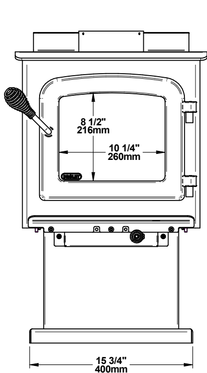
Figure 2: Vue de face
