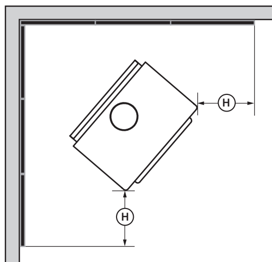
Figure 18: Dégagements pour l'écran de chaleur
